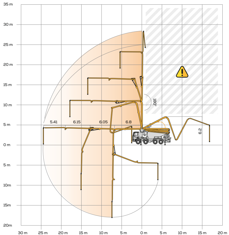
Verteilermast MK 28L-5"
